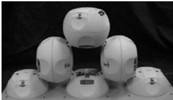
Rys. 8. Trzy prototypowe moduły ATRON na platformie testowej [24]
