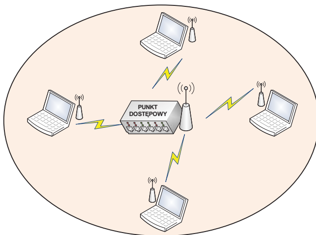
Rys. 2.4. Technologia sieci infrastrukturalnej BSS
