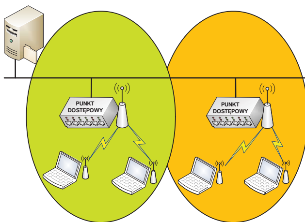
Rys. 2.5. Technologia sieci infrastrukturalnej ESS
