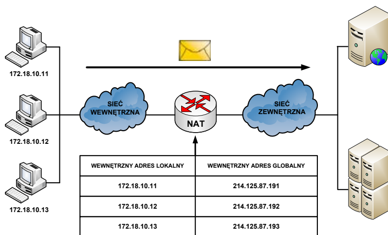
Rys. 2.3. Dynamiczna translacja NAT.
