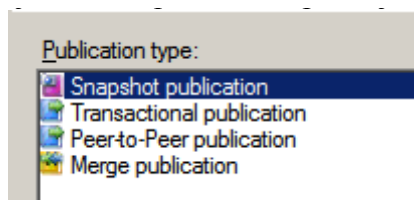
Rys.19. Typy replikacji
