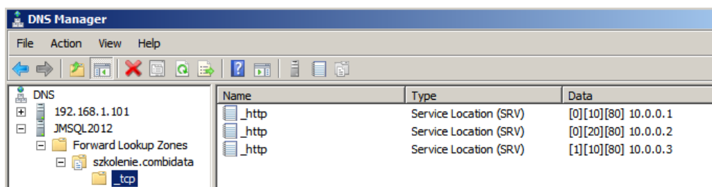
Rys.4. Rekordy SRV
