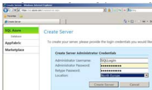
Rys.14. SQL Azure
