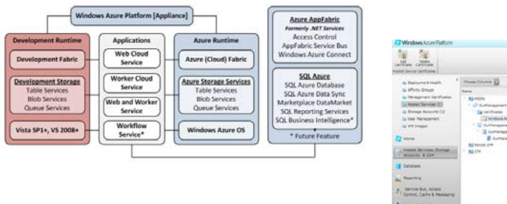
Rys. 12. Chmura obliczeniowa
